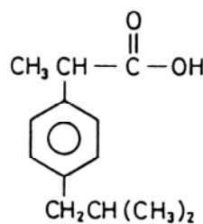
ibuprofène
