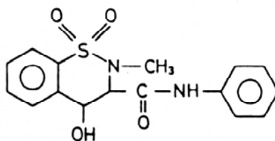
piroxicam
